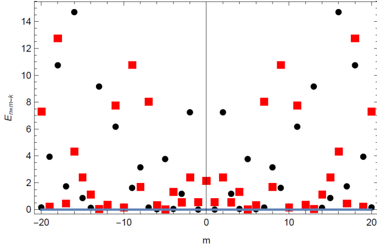
FIGURE 1 : Les 40 premiers niveaux d'énergie propres E_{n=m-k}^{k,i} du modèle donné dans l'équation (??) pour deux cas :
