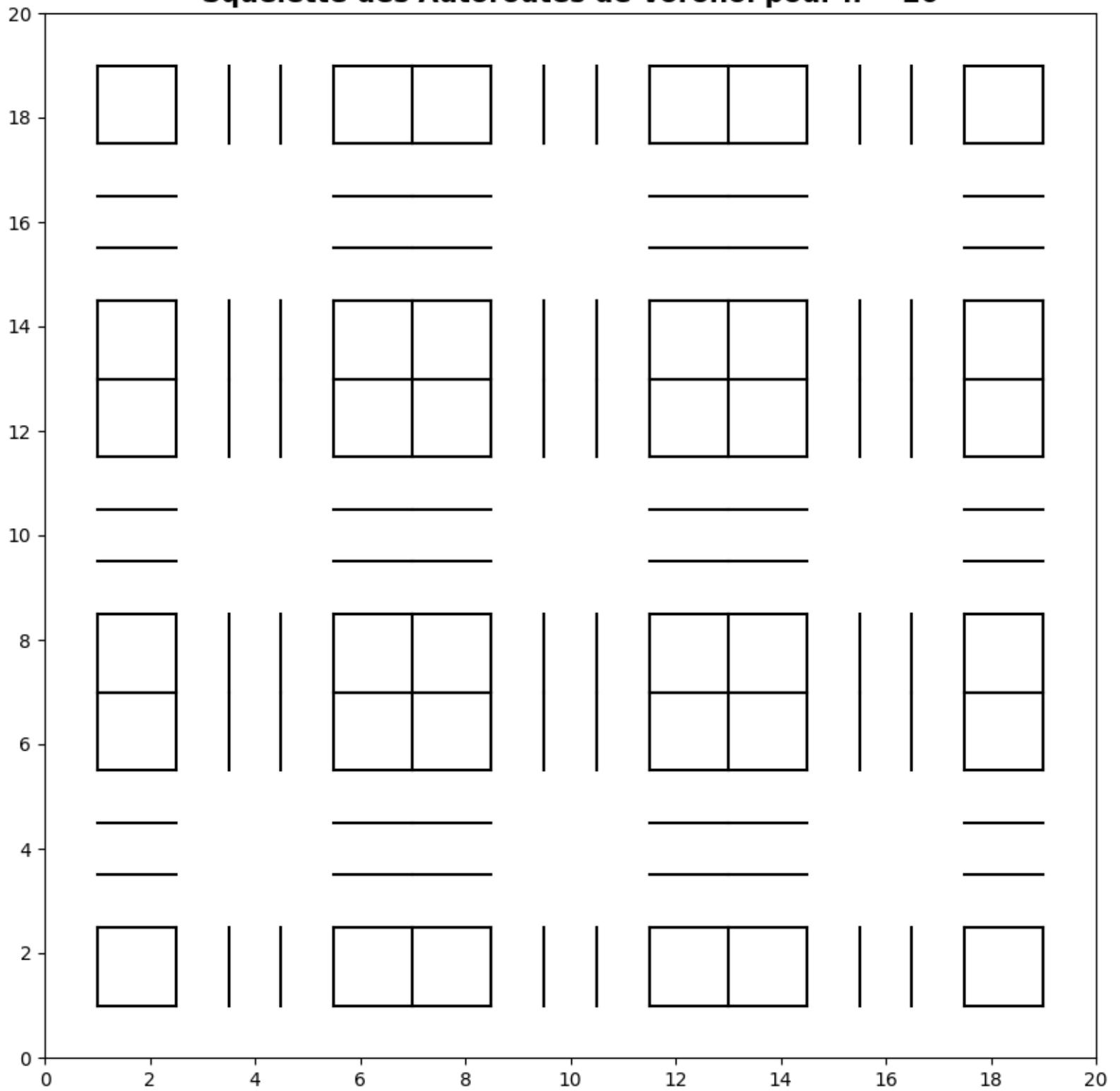
Squelette des Autoroutes de Voronoi pour n = 20
