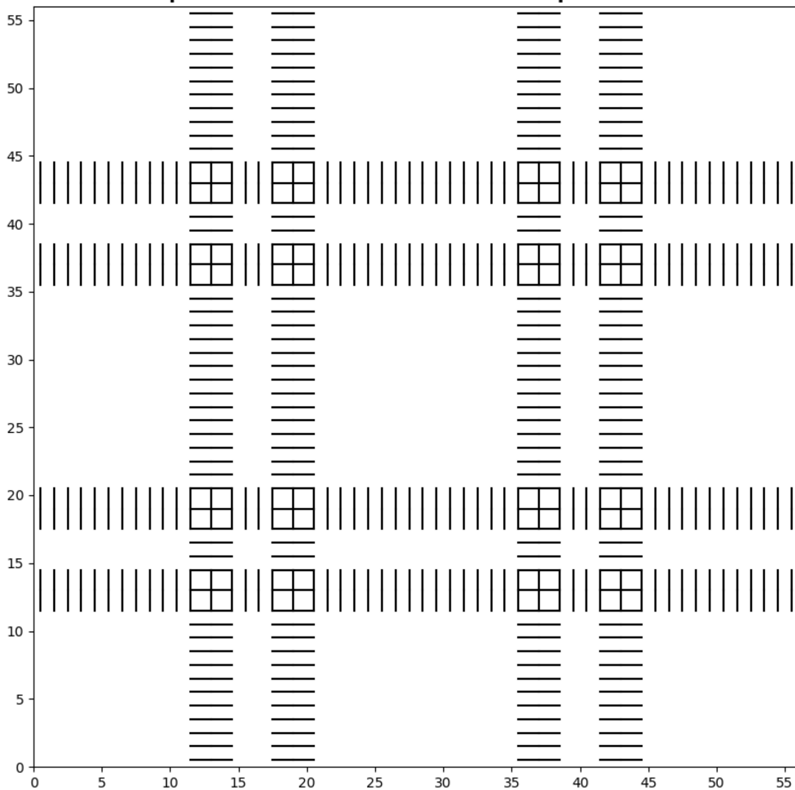
Squelette des Autoroutes de Voronoi pour n = 56
