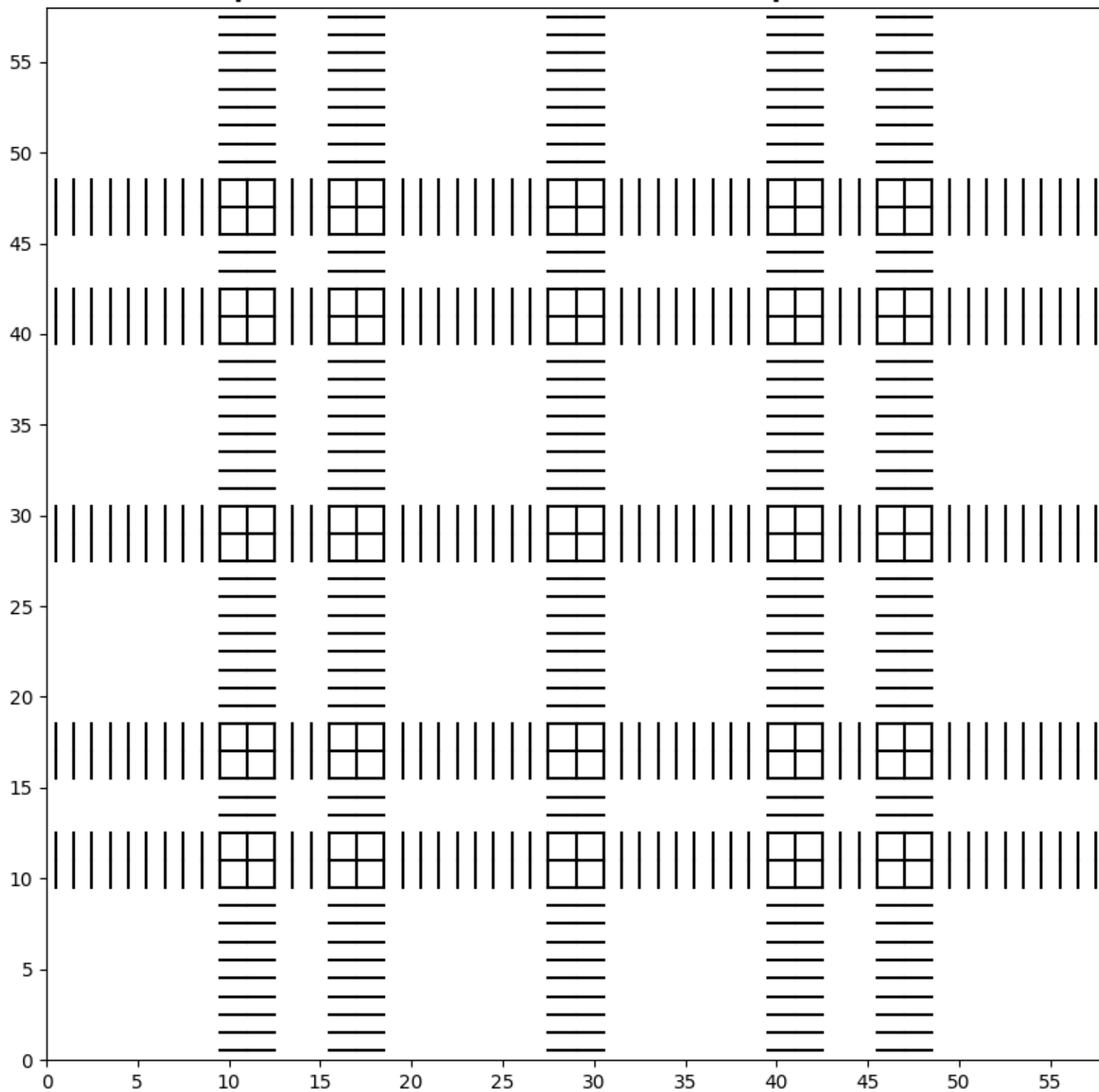
Squelette des Autoroutes de Voronoi pour n = 58
