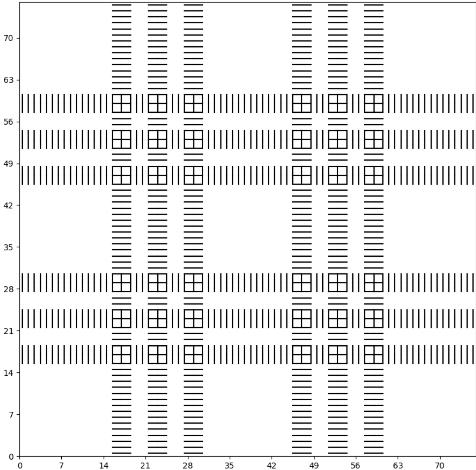
Squelette des Autoroutes de Voronoi pour n = 76
