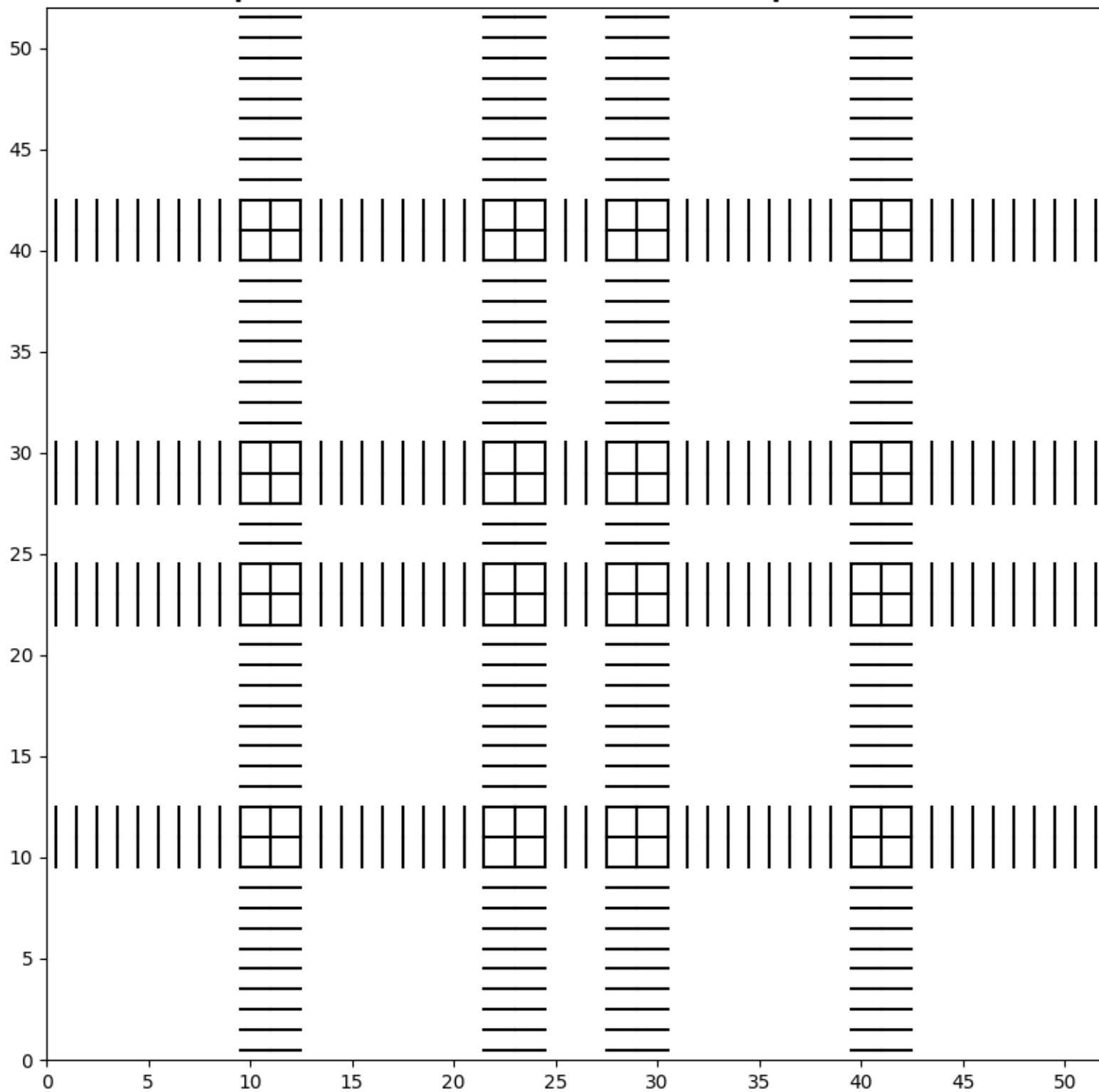
Squelette des Autoroutes de Voronoi pour n = 52
