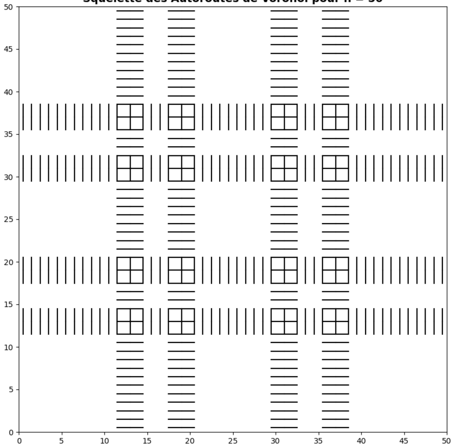
Squelette des Autoroutes de Voronoi pour n = 50
