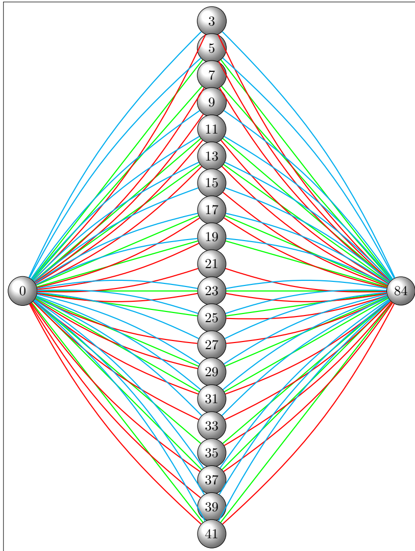
FIGURE 1 : graphe des incongruences pour n = 84
